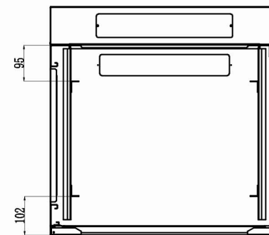
A-A Section
