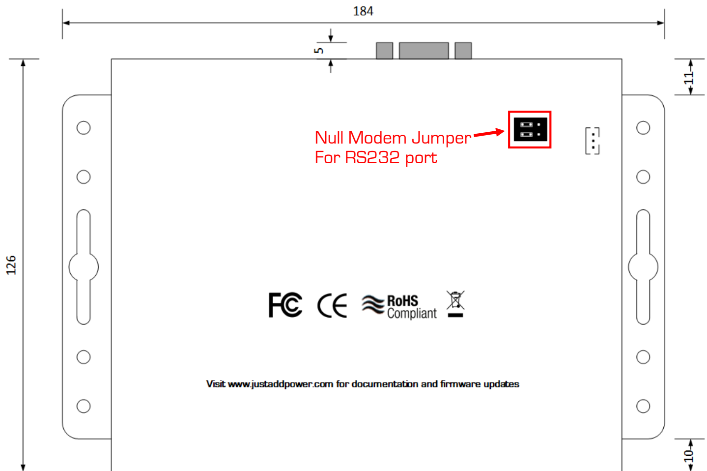
716VGA Bottom
